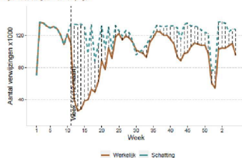
Figuur 10 Schatting stuwmeer verwijzingen
