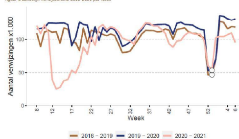
Figuur 2 Landelijk verwijzingsvolume 2018-2021 per week
